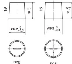
Anschlusspole 1
